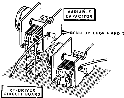
Detail 3-20A
