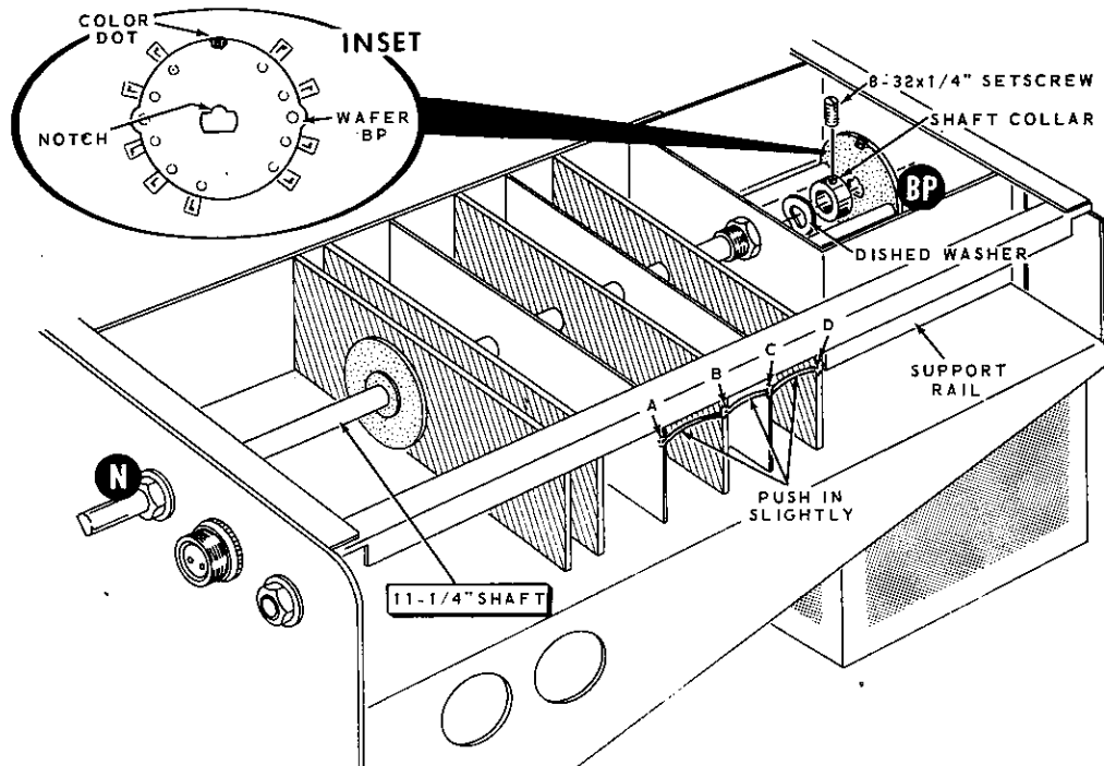
Detail 3-25E
