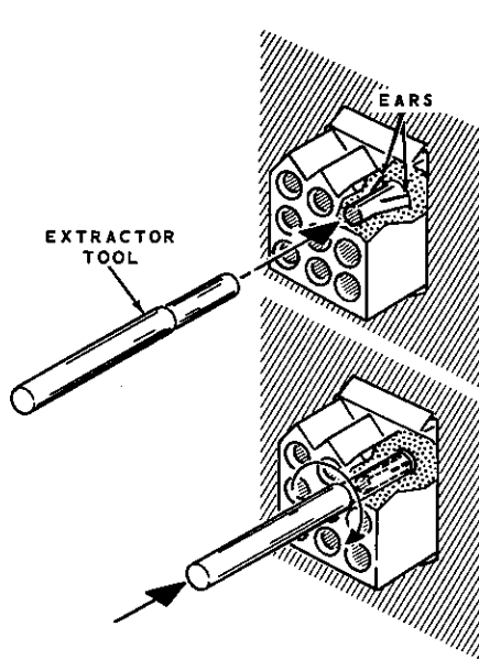
Detail 3-6E
