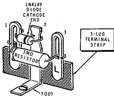
Detail 3-25B
