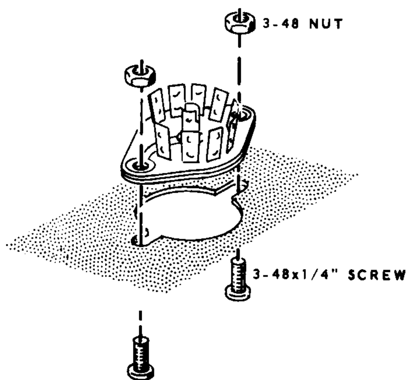
Detail 1A
